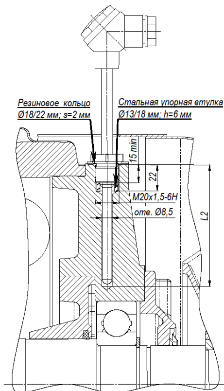
Рисунок К.5 – Варианты установки датчиков контроля температуры подшипников с собственной коробкой выводов
