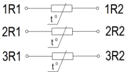
Рисунок А.3.1 – Типовая схема подключения термопреобразователей сопротивления обмотки Pt100
