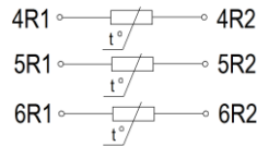
Рисунок А.3.2 - Типовая схема подключения термопреобразователей сопротивления обмотки Pt100
