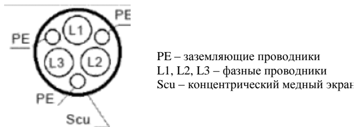
Рисунок В.3 – Пример экранированного кабеля
