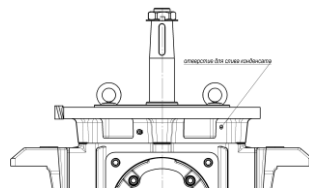
Рисунок 1 - Место положения сливного отверстия
