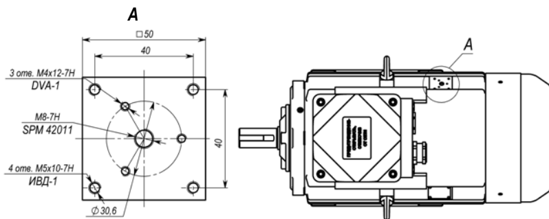
Рисунок Л.1- Место под установку вибродатчиков ИВД-1, DVA-1 и SPM 42011 на корпусе двигателя
