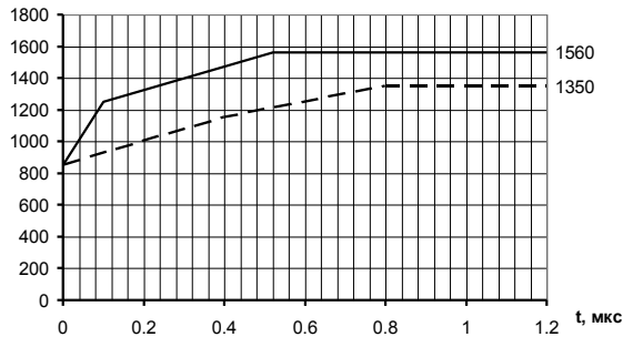
Рисунок В.1 - Зависимость допустимой амплитуды импульса от времени
