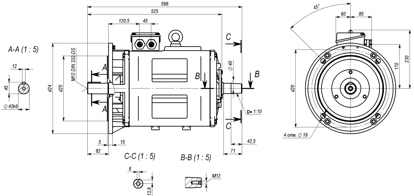
Габаритный чертеж Dimension drawing
